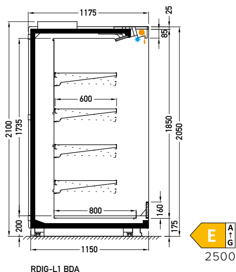
RDIG-L1 BDA
