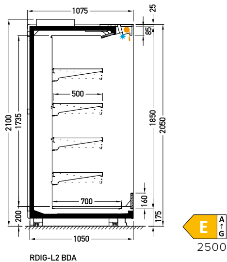
RDIG-L2 BDA
